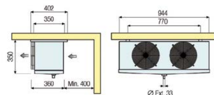
TN BT 022 016
