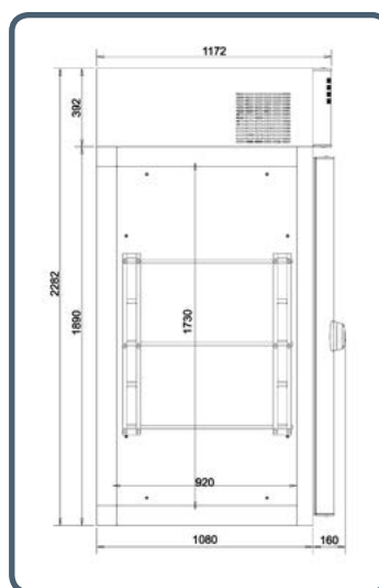
ESQ. DIMENSIONES
