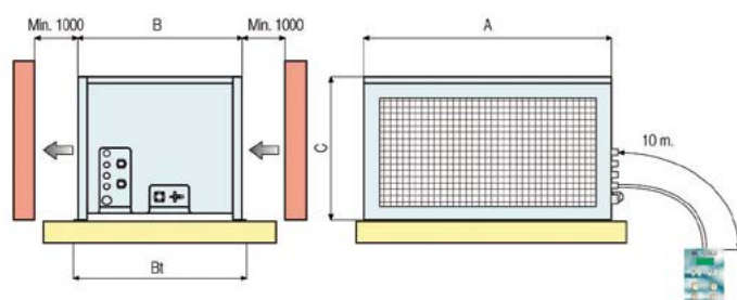
CONDENSADORA - Unidad exterior
