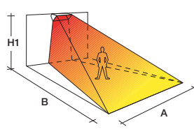
Esquema de Instalación y área radiada
