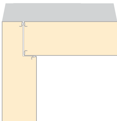
Opción 1: Sistema de unión panel vertical-techo Sistema tipo IV
