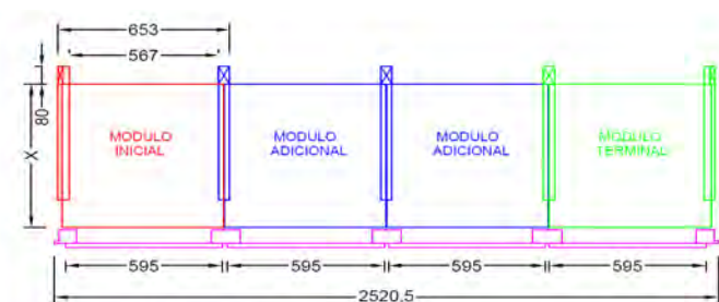
COTAS BLOQUE DE 4 PUERTAS DE CRISTAL DIM PUERTA 595
