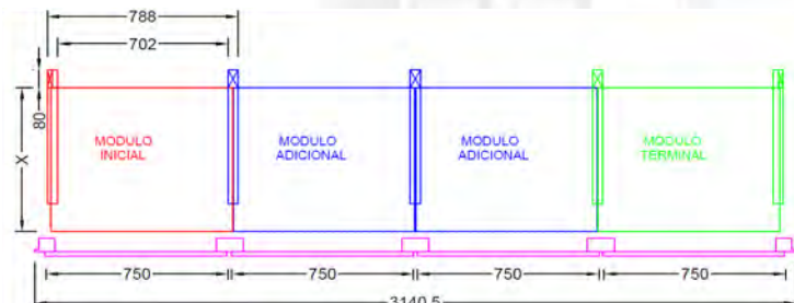
COTAS BLOQUE DE 4 PUERTAS DE CRISTAL DIM PUERTA 750
